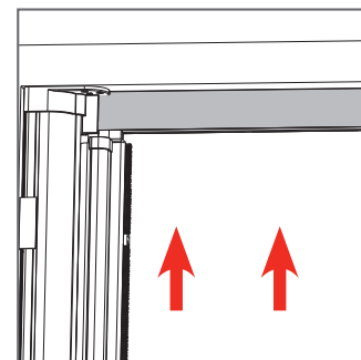
5 Inserire la guida superiore.
