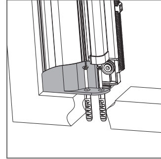
3 Procedere con il fissaggio della coprestata inferiore e superiore.
