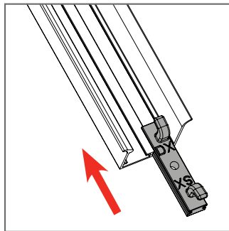
4 Inserire gli agganci Dual Hook e i fermoguida nella guida di riscontro laterale.
