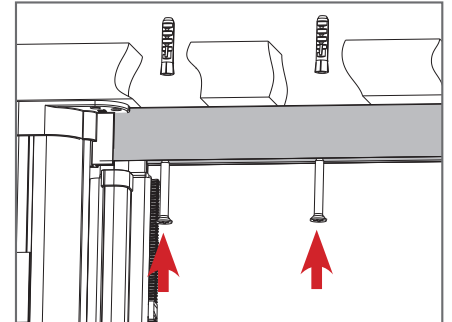
8 Fissare la guida superiore.
