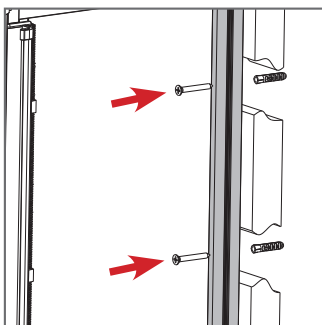
9 Fissare il profilo riscontro laterale.
