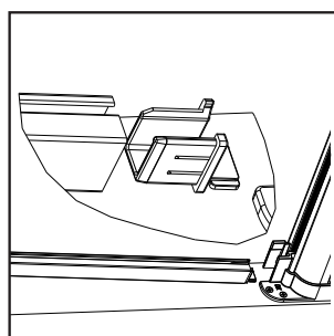
15 Inserire la guida inferiore di destra nella copritestata.
