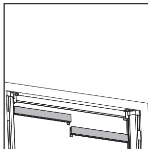
7 Inserire compensatore di sinistra e fissarlo.
