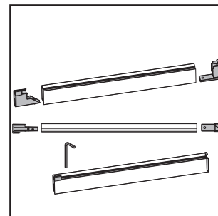
8 Inserire l'aggancio guida bassa, rispettando il verso (la parte sottile verso esterno).
