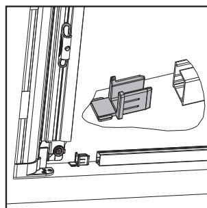
11 Inserire piedino guida inferiore.
