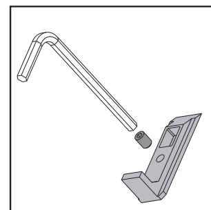
12 Avvitare il grano nel fermo cricchetto guida bassa.
