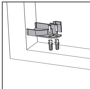
1 Fissare la copritestata inferiore di sinistra.
