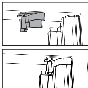
6 Inserire il copritestata superiore di destra e fissarlo.
