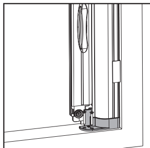
5 Dopo aver fissato il copritestata inferiore di destra inserire il cassonetto di destra.
