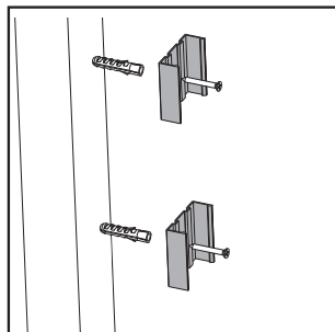
2 Fissare le staffe.
