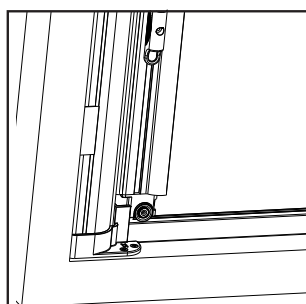
13 Inserire la guida inferiore di sinistra nella copritestata.
