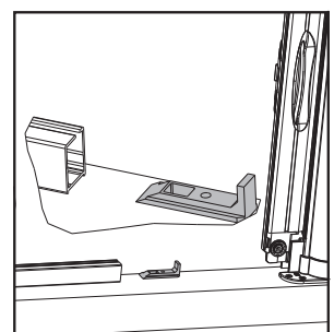
14 Inserire il fermo cricchetto nella guida bassa (lato cassonetto con cricchetto).
