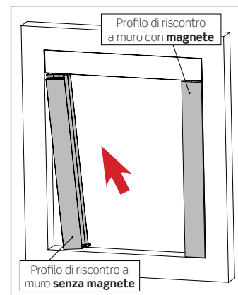
9 Posizionare i riscontri nel vano.
