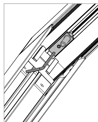
12 Posizionare la baionetta in battuta con il tappo (il dentino evidenziato funge da dima) e solo dopo fissare con i grani.
