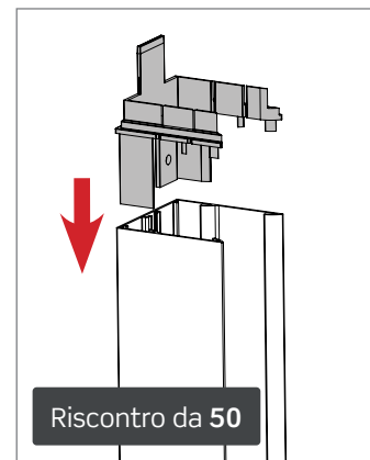
7 Inserire i tappi superiori nei riscontri laterali.
